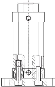
Крепление снизу
